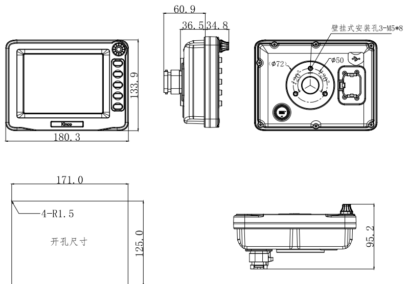
CZ6尺寸图 单位:mm
